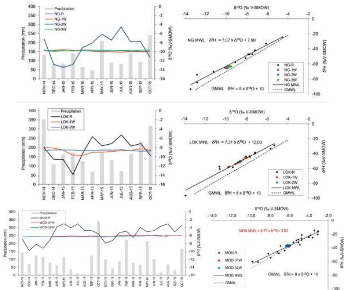
Slika 3. Mjesečne varijacije izotopnog sastava ( \delta^2\text{H} i \delta^{18}\text{O} ) kišnice i prokapsnica, te usporedba lokalnih s globalnom linijom meteorske vode (GMWL)
